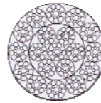
18x9S + WSC
