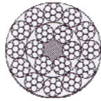
18x7 + FC
