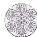
6x31WS + IWRC
