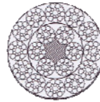
18x19S + FC
